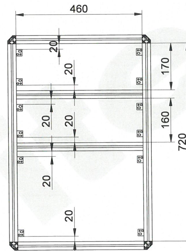
Schnitt B-B
