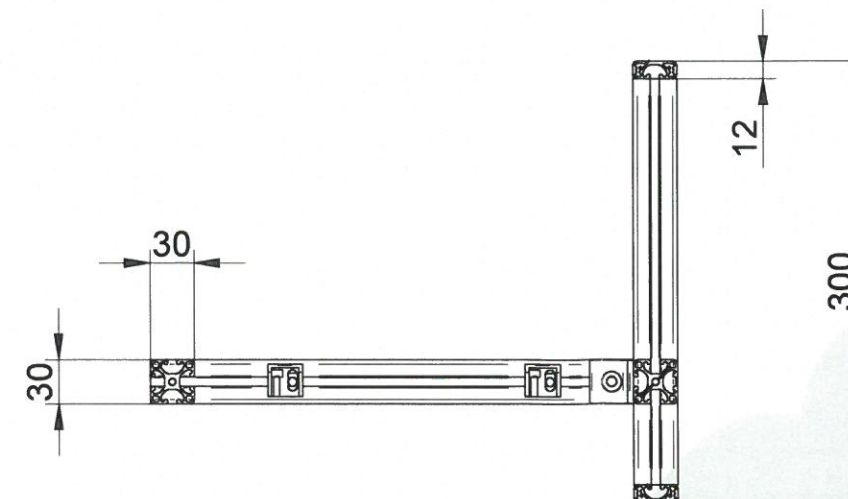
Schnitt G-G
